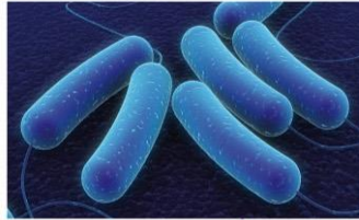
▼ Bacteria 0,3 – 20 \mu\text{m}
