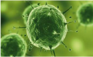
▼ Viruses 0,003 – 0,05 \mu\text{m}
